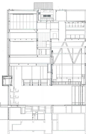
Sección longitudinal / Longitudinal section
