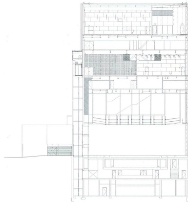
Sección transversal / Cross section
