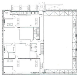
Planta cuarta / Fourth floor plan
